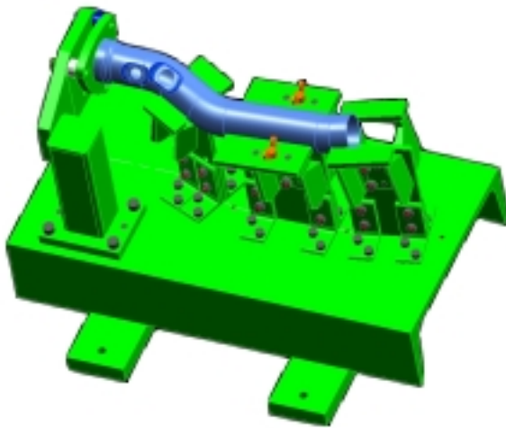
Beispiel: PKW-Abgasanlage
